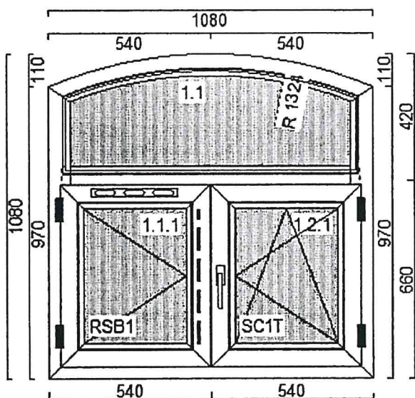
Szerokość 1080mm x Wysokość 1080mm
