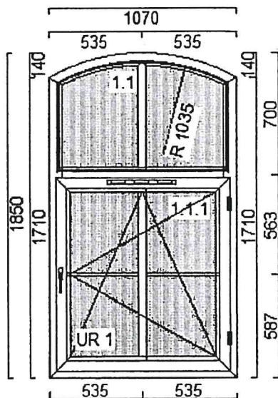
Szerokość 1070mm x Wysokość 1850mm
