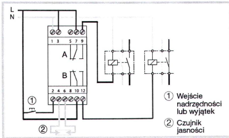
Rysunek 2: Schemat podłączeń przełącznika EGN200 (2 wyjścia)
