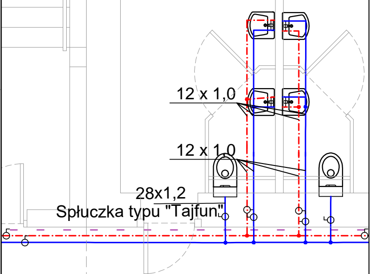
Przykładowy węzeł wody użytkowej
